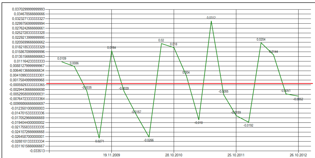
Abbildung 2 - Die positiven und negativen Abweichungen mehrerer 10 V - Messungen über die Jahre
